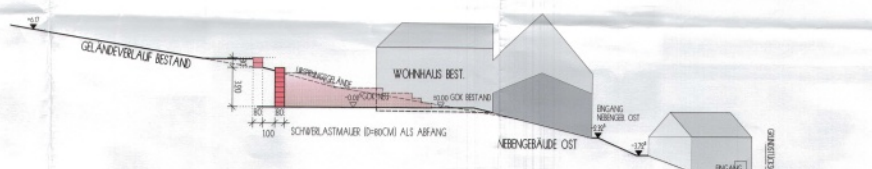
SNITT B-B M. 1:200
